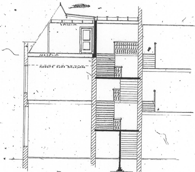
DOORSNED E. C. D.
