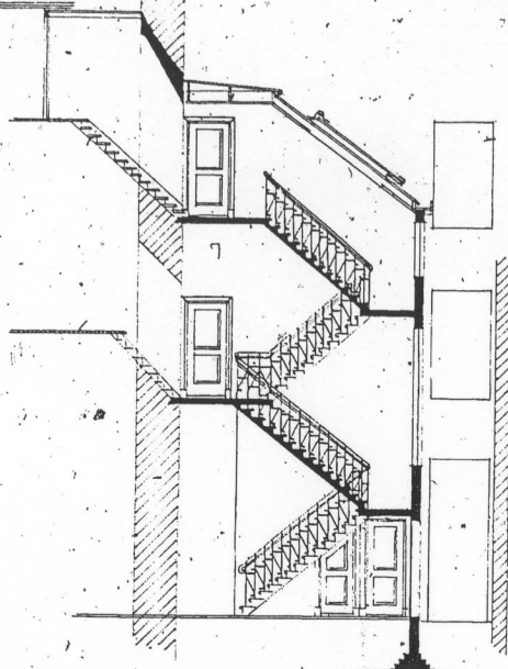
DOORSNED E. A. D.
